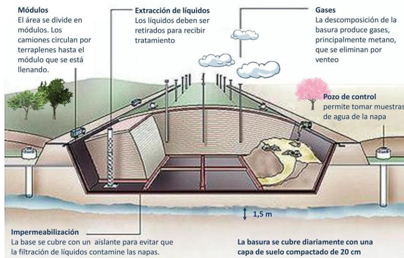
Torri, SI. 2017. Corte de un relleno sanitario. ¿Qué es un relleno sanitario? Publicación on-line del Centro de Estudios y Desarrollo de Políticas Públicas, CECEPP, http://cedepp.org.ar/?p=381
